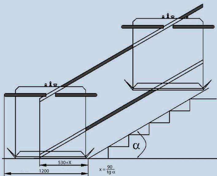
Przestrzeń niezbędna do zainstalowania platformy
