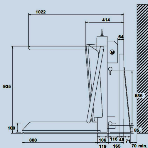
Mocowanie platformy do słupków
