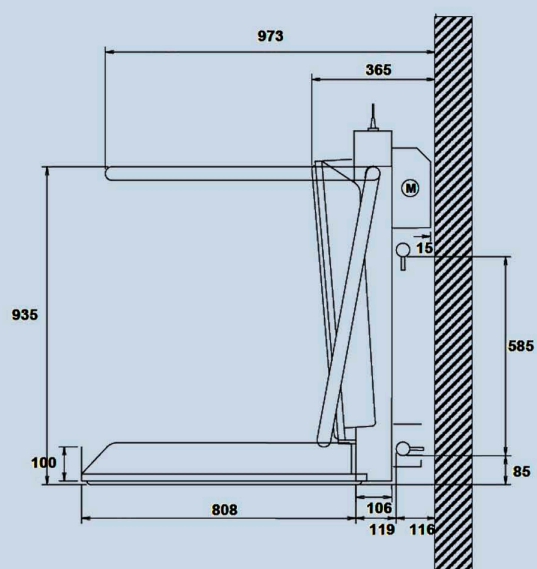
Mocowanie platformy do ściany
